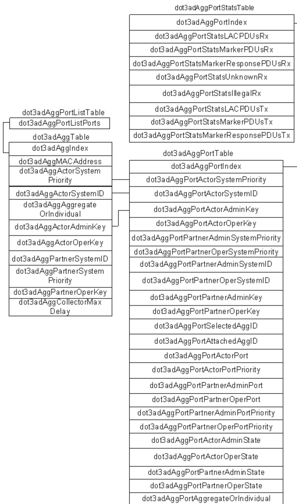
图 152-1 LACP-MIB Table 的表间关系图
